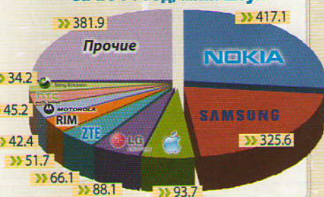
Продажи телефонов за 2011 год, млн. штук
