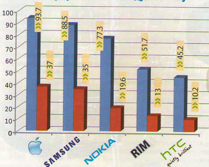
Ведущие производители на рынке смартфонов в 2011 году, млн. штук
