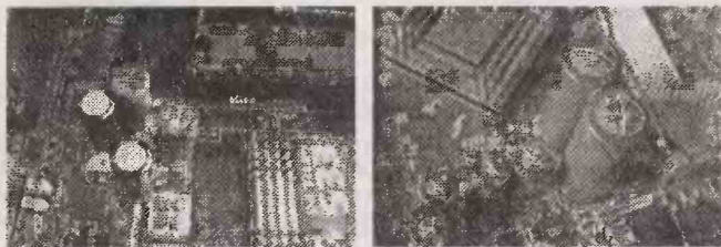
Неисправный конденсатор (справа) легко отличить от исправного по характерному «вспучиванию» в верхней части корпуса
