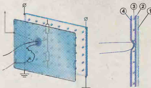
Принцип действия 4- и 5-проводных резистивных сенсорных экранов
