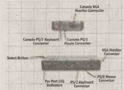
З допомогою KVM перемикають сигнали монітора, клавіатури та миші, але є засоби для звука та USB
