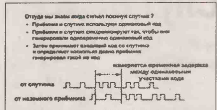
Рис. 3 Сигнал от спутника добирается до Земли не мгновенно. Для определения этого времени и придумана система с генерацией псевдослучайного кода
