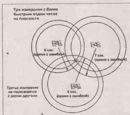
Рис. 5 В случае ошибки по времени на стороне приемника система из трех спутников тоже дает точные данные
