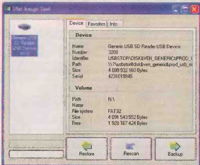
Рис. 2: Главное окно программы USB Image Tool
