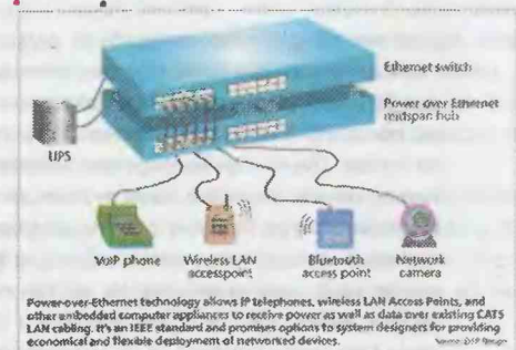
Среди PoE-устройств, кроме упомянутых в статье, можно обнаружить VoIP-телефоны и точки доступа Bluetooth
