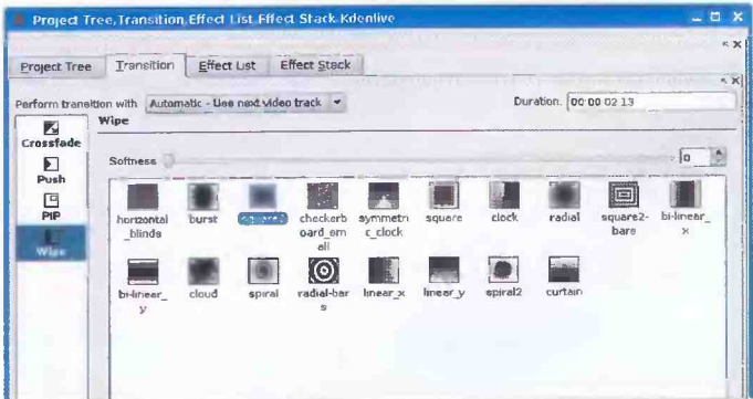
Рис. 2 Эффекты перехода
