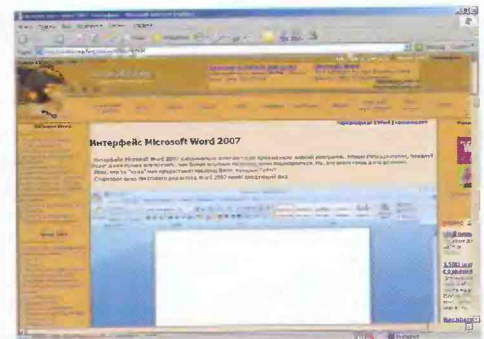
Рис. 3 Изучаем интерфейс
