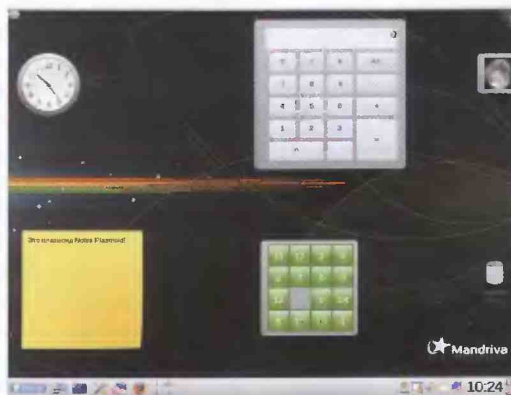
Рис. 3 Четвертый KDE со своими плазмоидами
