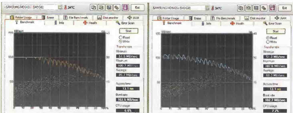
Рис. 8 «Особенная» сервосистема проявляет себя в виде зубцов на графиках скорости HD642JJ. Хотя при записи первые 30% идут ровные 100 МБ/с
