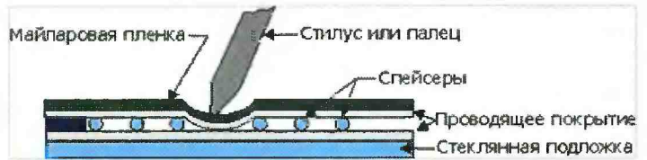
Рис. 6 Устройство резистивного тацскрина — просто, дешево и надежно
