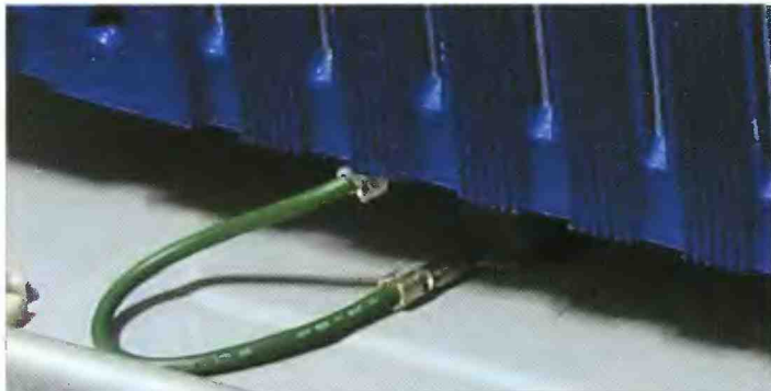
Рис. 8 Вот так выглядит правильно установленная клемма заземления
