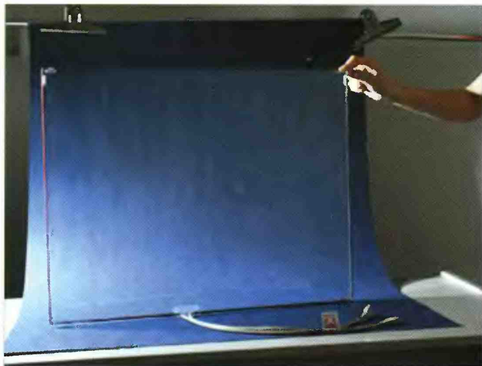
Рис. 10 Ультразвуковые тачскрины могут иметь довольно внушительные размеры
