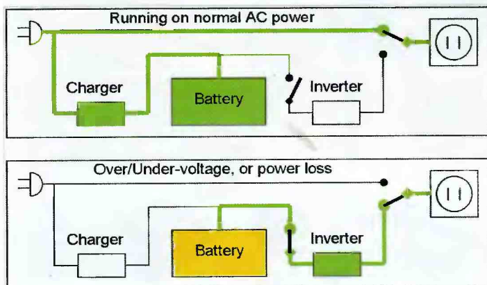
Работа ИБП пассивного типа в нормальном режиме и в автономном
