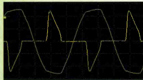
Зелёная линия — напряжение, подаваемое на компьютерный БП, а жёлтая — ток, который БП использует. Ток явно не синусоидный...
