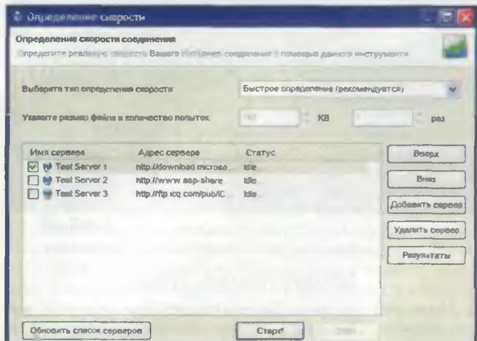
Рис.3 Измеритель скорости интернет-соединения
