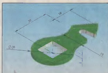
Рис.9 Крючок замка
